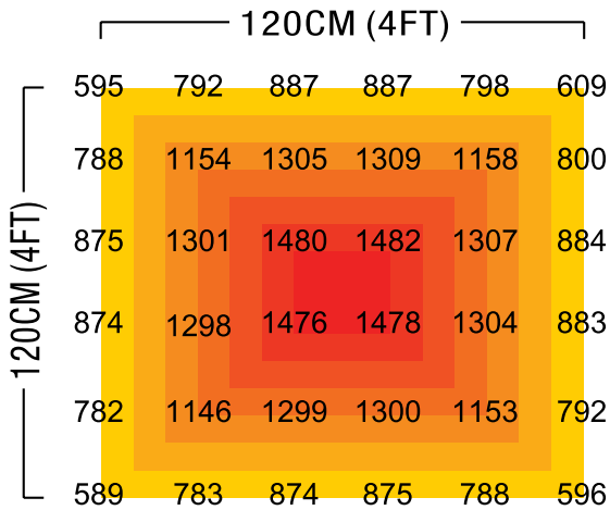
Height of 12" / 30CM PAR Distribution
