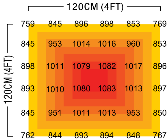
Height of 31" / 80CM PAR Distribution
